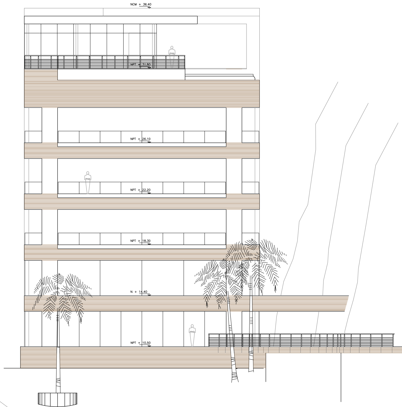
elevación norte esc : 1:75
